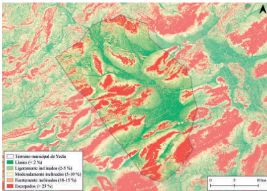
Figura 2. - Pendientes y formas del relieve en el término municipal de Yecla
